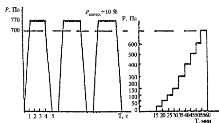
Рисунок 5 — Пример построения графиков испытаний оконных блоков на водопроницаемость для конечного контрольного давления 300 и 700 Па
