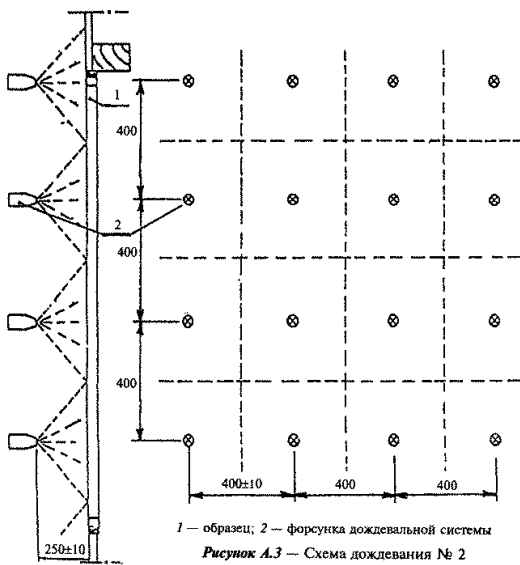
Рисунок А.3 — Схема дождевания № 2
