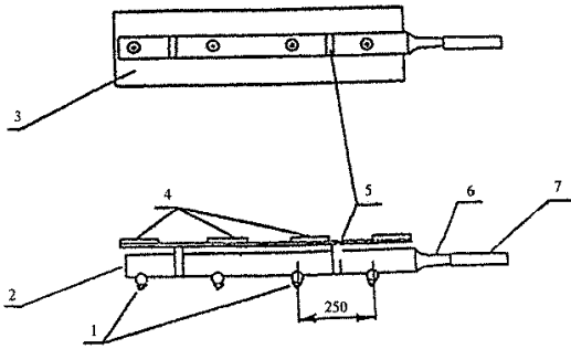
Рисунок А.2 — Элемент дождевального оборудования (распределительная трубка)
