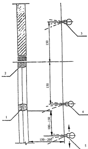
1 — образец, верхний брусок коробки, 2 — образец, горизонтальный импост, 3 — верхний неподвижный ряд форсунок; 4 — второй сверху неподвижный ряд форсунок; 5 — дополнительный ряд форсунок
